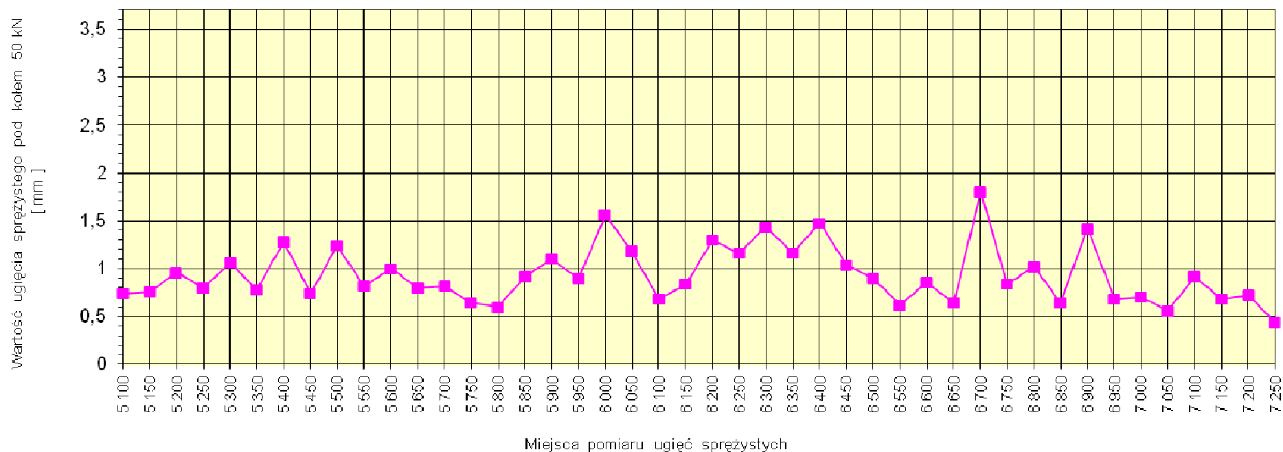
Rys. 1b Pomiary ugięć sprężystych - drogi 1538D i 1466D - od km 5+100 do km 7+250
