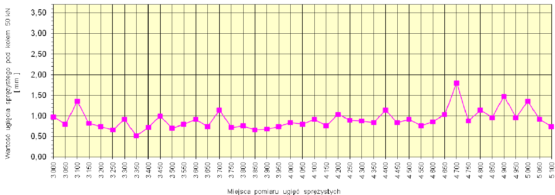
Rys. 1a Pomiary ugięć sprężystych - drogi 1538D i 1466D - od km 3+000 do km 5+100
